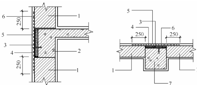
图 5.2.5-2 梁、柱与墙体交接处保温处理的构造做法示意
