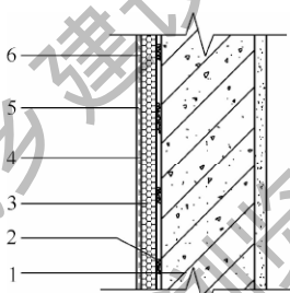
图 5.2.5-1 热桥部位保温处理的基本构造示意
