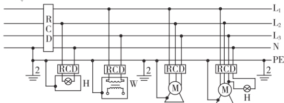
图 A. 0.2 外电路直接供电的局部 TN-S 系统
